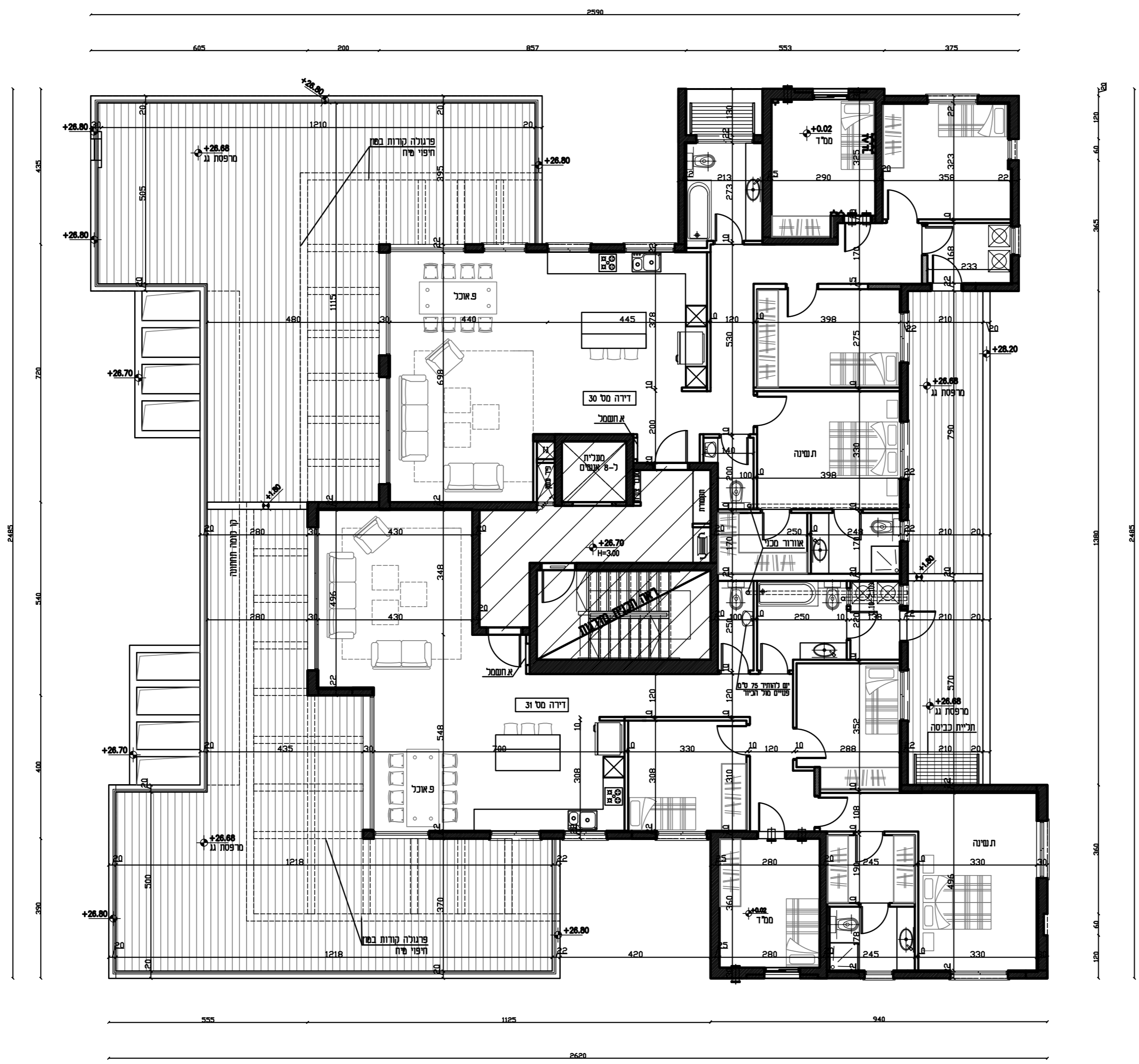
תכנית קומה ח' קנ"מ 1:100
